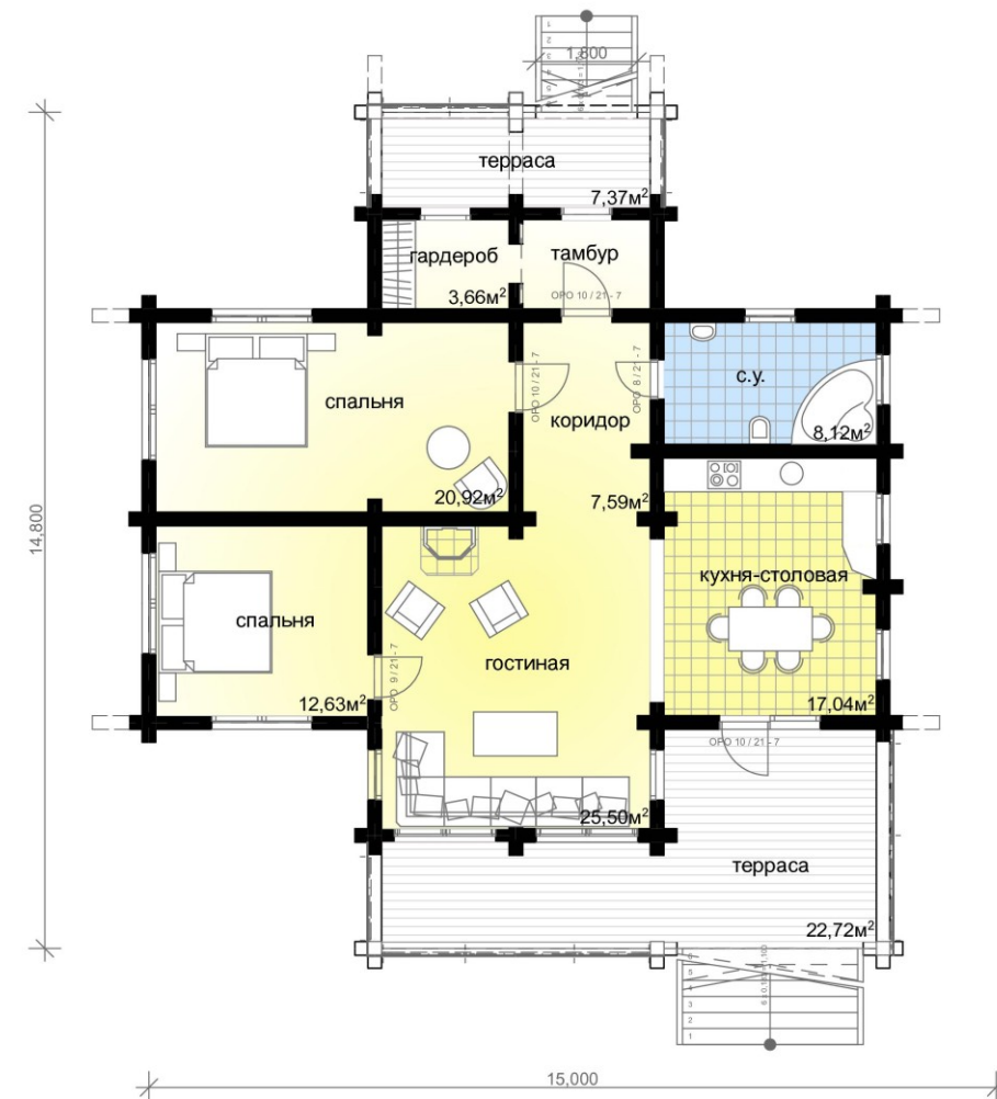
План 1-го этажа
