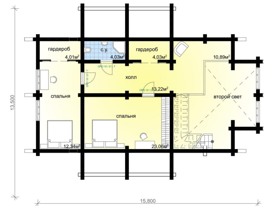
План 2-го этажа
